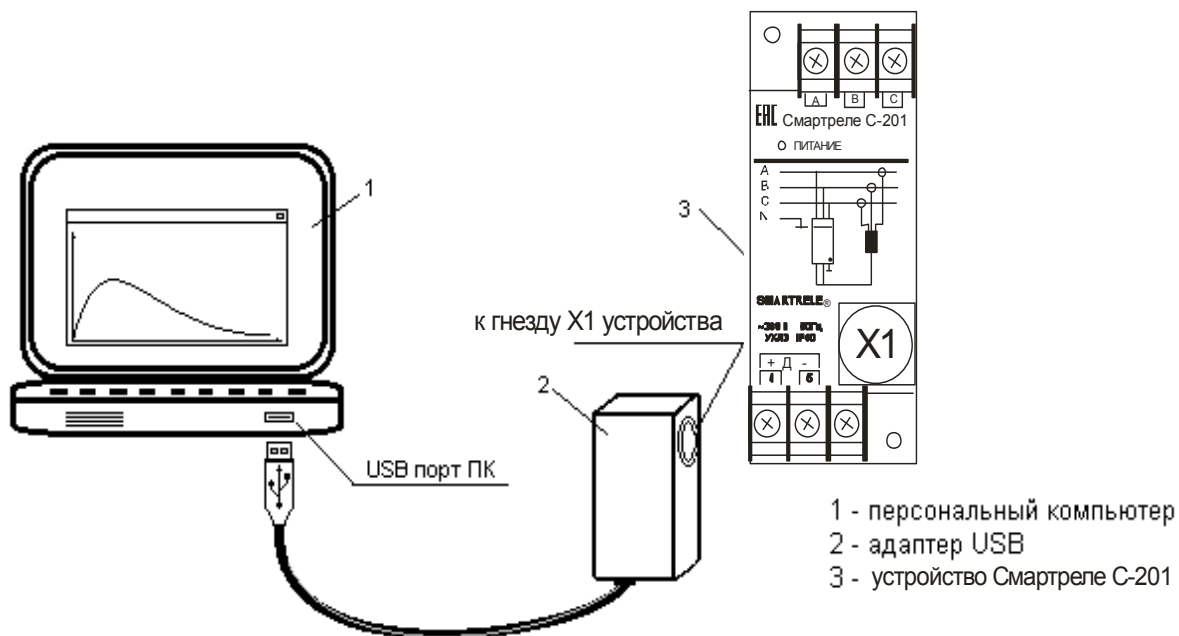
Рисунок 5 - соединение устройства СМАРТРЕЛЕ C-201 с ПК посредством Адаптера USB
