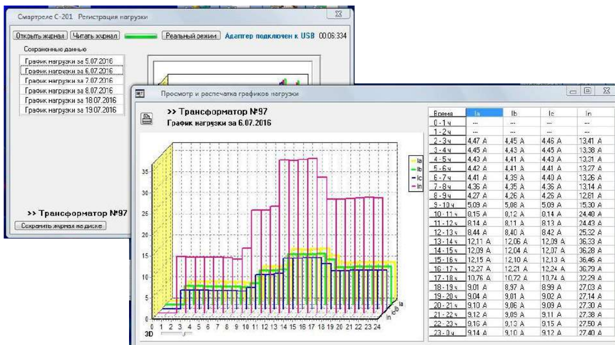
Рисунок 6 - отображение суточного графика нагрузки объекта на экране ПК
